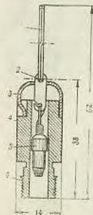
Рис. 55. Терочный воспламенитель: 1 — вытяжное кольцо; 2 — серва; 3 — колпачок; 4 — корпус; 5 — терочный элемент; 6 — выходящая часть.
