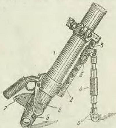
Рис. 82. Ствол с подъемным механизмом 50-мм германского миномета: 1 — ствол; 2 — трубка; 3 — втулка; 4 — стальная муфта подъемного механизма; 5 — англо; 6 — спусковая рукоятка стреляющего приспособления; 7 — сектор; 8 — стоп; 9 — чека
