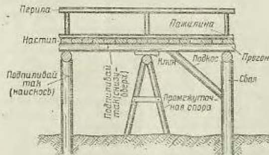
Рис. 36. Разрушение деревянного моста вручную
