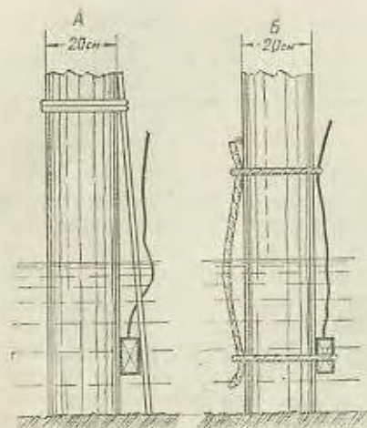
Рис. 38. Перебивание свай рядами, расположенными под водой;
