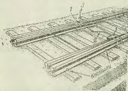
Рис. 24. Расположение зарядов для подрывания стрелок: 1 — заряд; 2 — детонирующий шнур; 3 — зажигательная трубка
