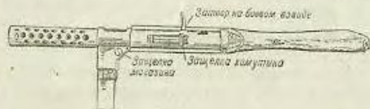
Рис. 60. Пистолет-пулемет 28/П заряженный
